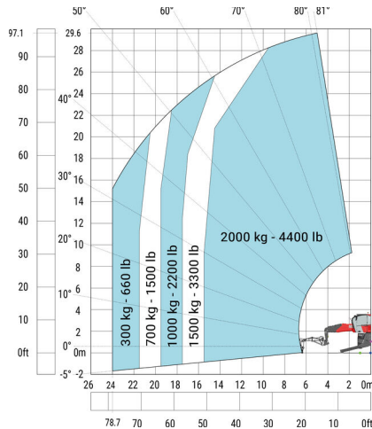
Drehung mit abgelaassenen Stützen mit 3D positiv/negativ
