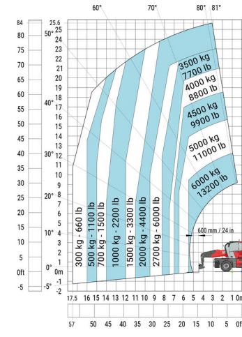
Drehung mit abgelaassenen Stützen und 2 to jib (Metrisch)
